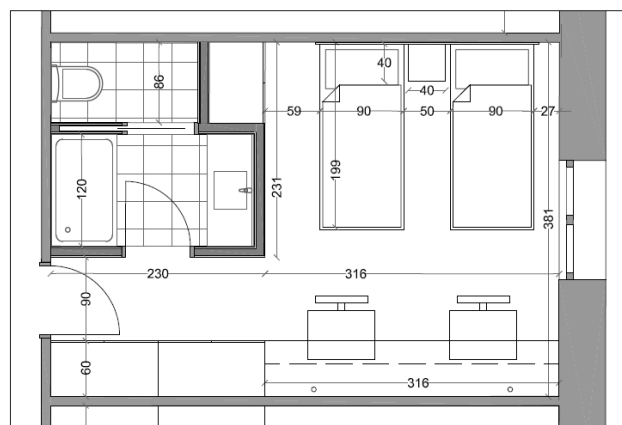
DORMITORIO TIPO E1/50
